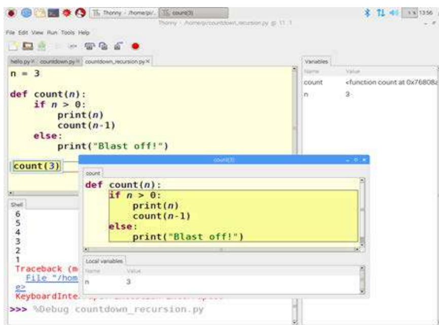
Рис. 93. Интерфейс программного продукта IDE Thonny
