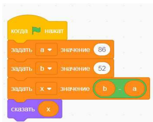
Рис. 118. Вид программы
