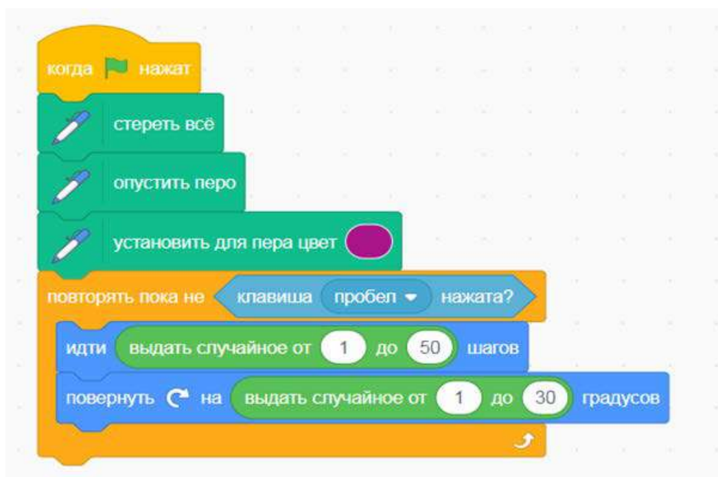
Рис. 130. Вид программы
